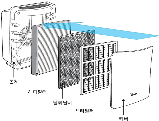
필터 장착 순서
