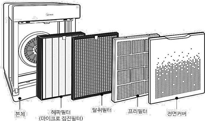
필터 교체 방법 (기기의 전원을 끈 후 교체해 주세요.)
