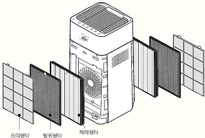
필터 교체 방법 (기기의 전원을 끈 후 교체해 주세요)
